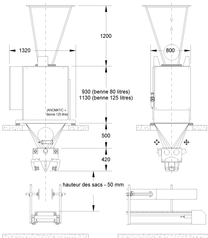
"JANOMATIC G/60-6" avec bouche d'ensachage à bec de canard pour ensachage de produits granuleux.
